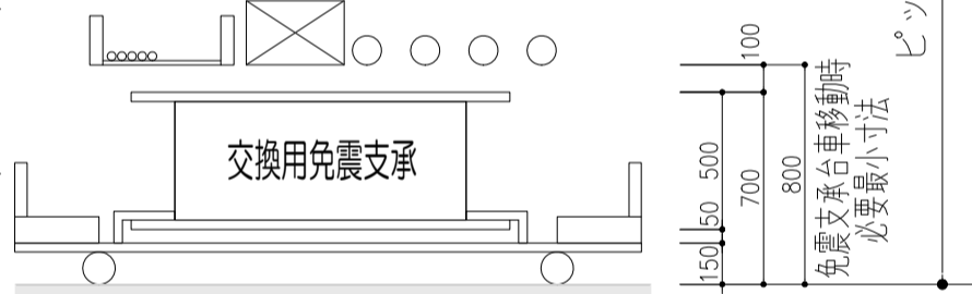
免震メンテナンス動線上部クリアランス詳細 1/30
