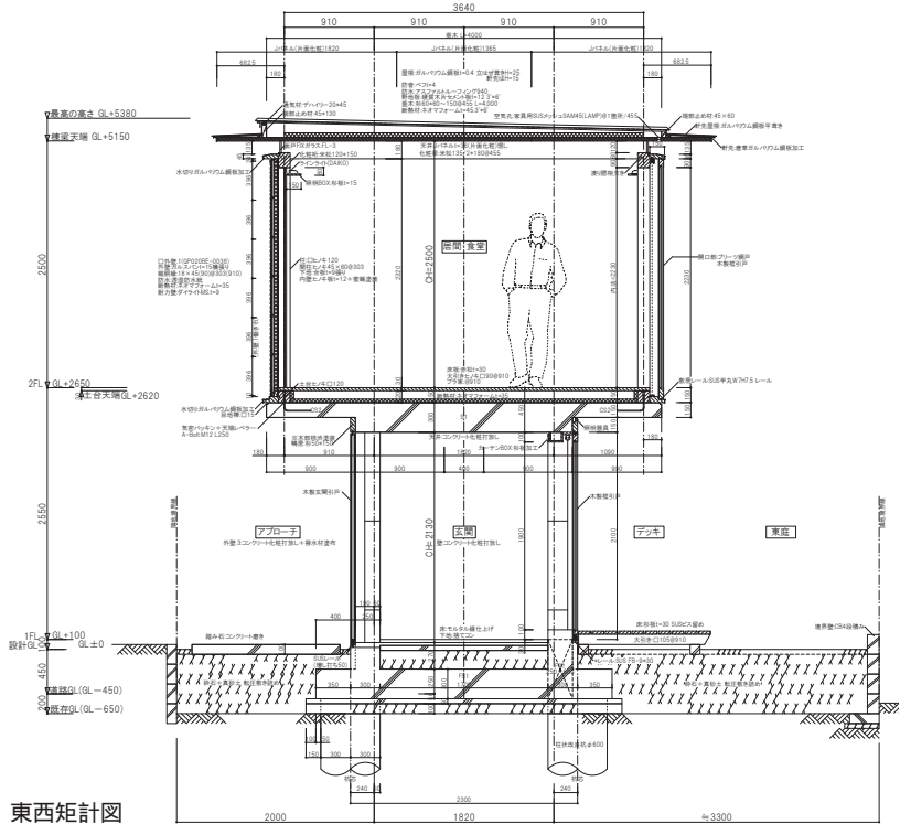
東西矩計図
