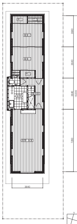
2階平面図
